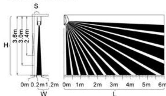
墙壁安装探测区域图
